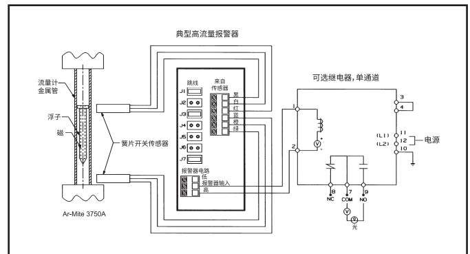
簧片开关布线图
